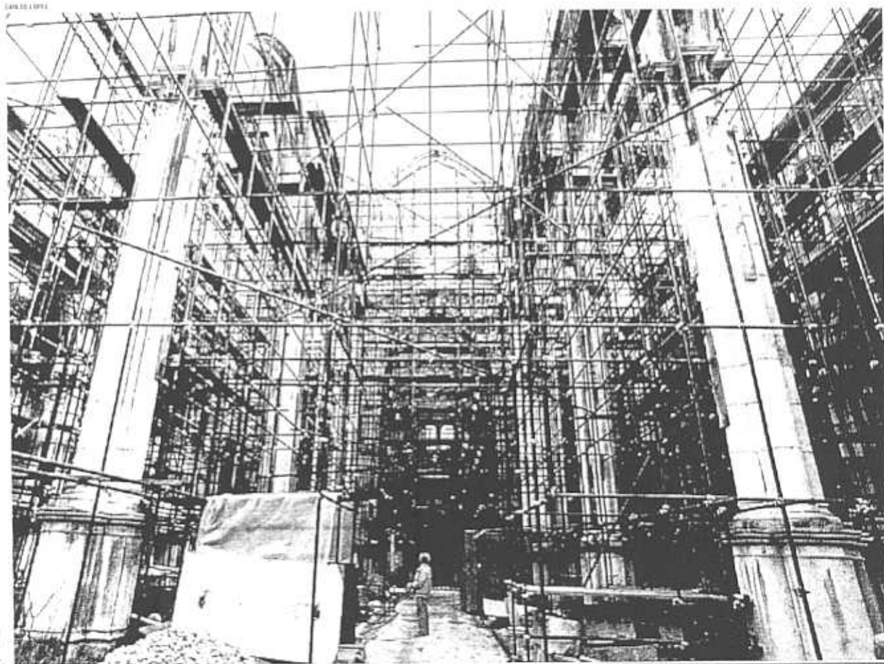
O escoramento da nave está a ser retirado, mas "revelou-se desnecessário" durante a construção do túnel, sustenta o Metropolitano
